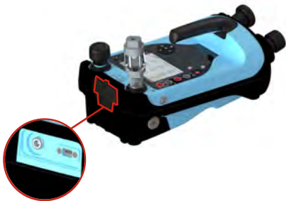
Figur 1. DPI610E-opladningsport
