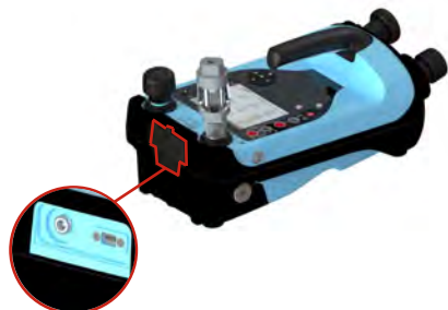
Figur 1: DPI610E laddningsuttag
