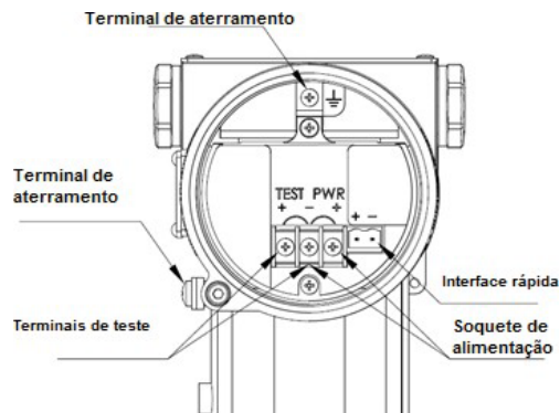
Figura 7 – Identificação dos terminais da borneira
