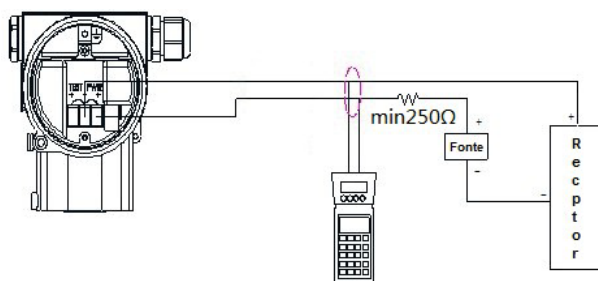
Figura 4 – Ligação elétrica
