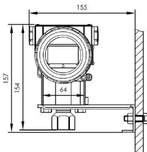
Figura 23 – Montagem em parede e na vertical – RP2002 e RP2003
