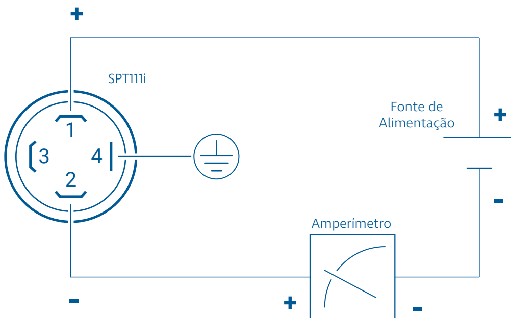
Figura 4 - Esquema de ligação 4...20 mA do transmissor SPT111i
