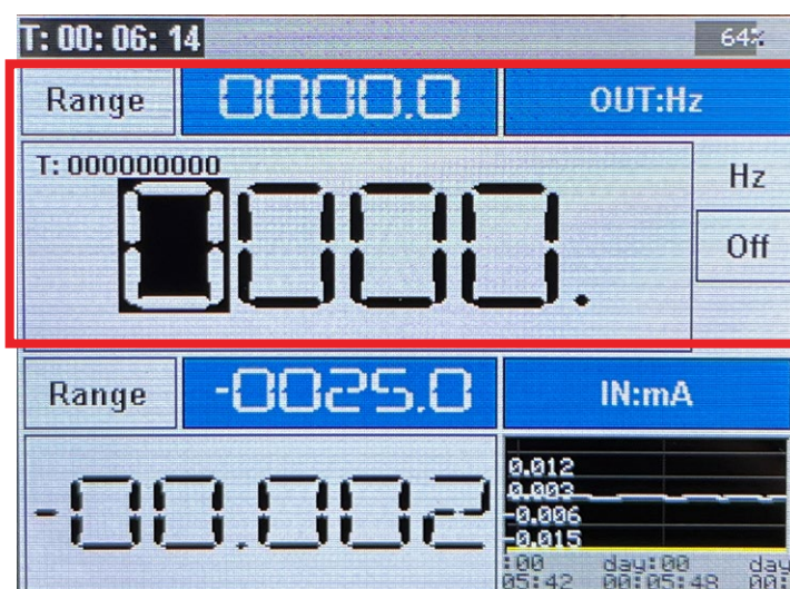
Figura 36 - Tela no modo de geração de frequência
