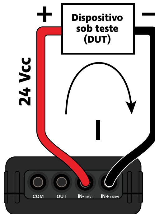
Figura 15 - Forma de conexão do SLC100+ para medição ativa de corrente
