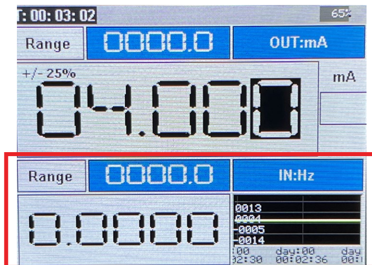
Figura 18 - Tela no modo de medição de frequência
