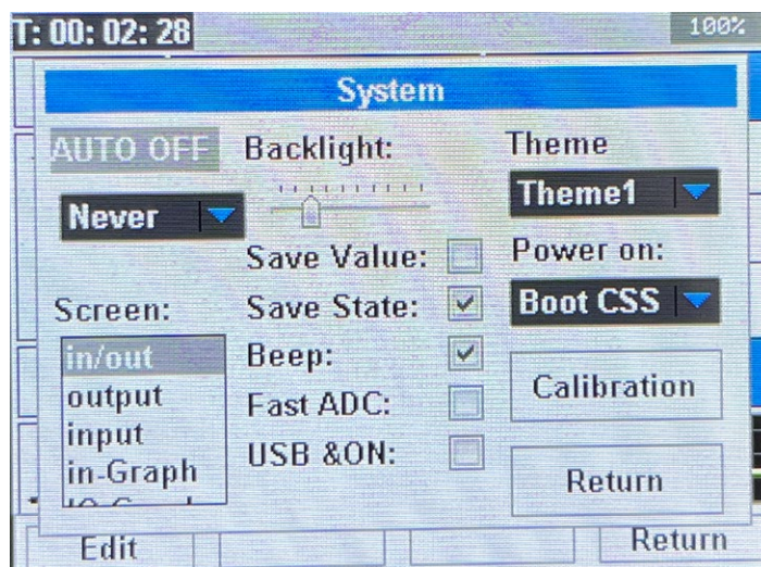
Figura 56 - Tela de configurações gerais do SLC100+
