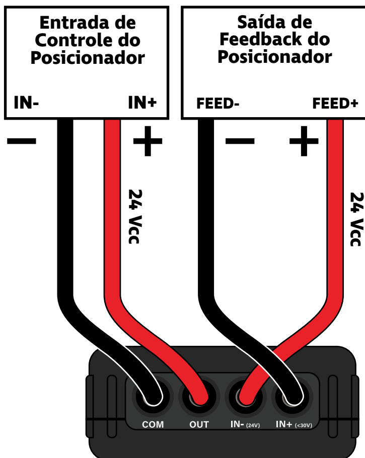
Figura 51 - Diagrama de conexão para teste de posicionadores pneumáticos
