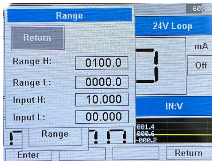
Figura 8 - Tela de configuração da faixa da entrada elétrica
