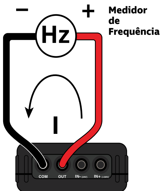
Figura 38 - Forma de conexão do SLC100+ para geração de frequência (modo Level)
