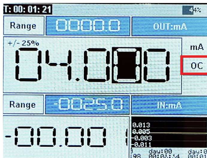
Figura 29 - Indicação de falha na geração ativa de corrente
