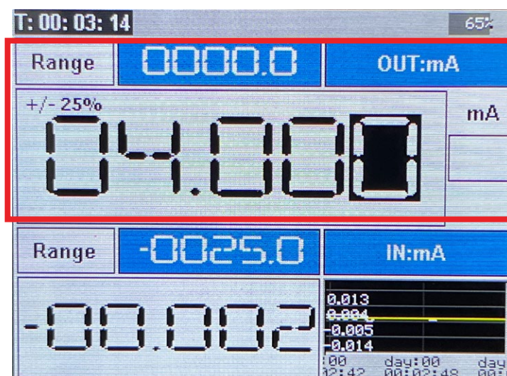
Figura 27 - Tela no modo de geração de corrente
