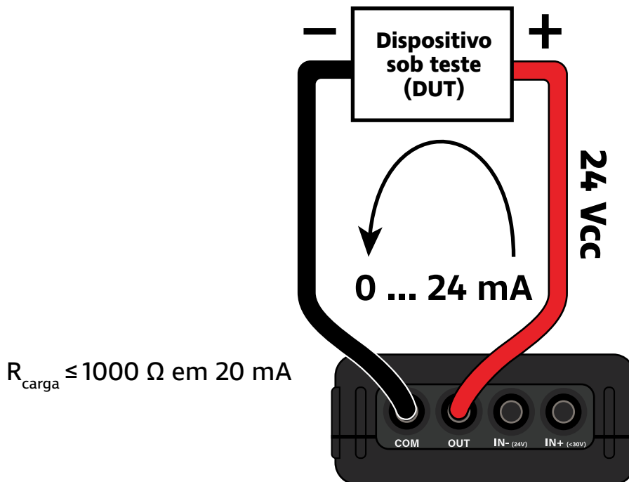
Figura 28 - Forma de conexão do SLC100+ para geração ativa de corrente
