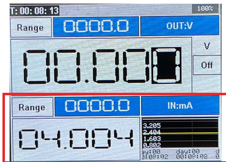
Figura 10 - Tela no modo de medição de corrente
