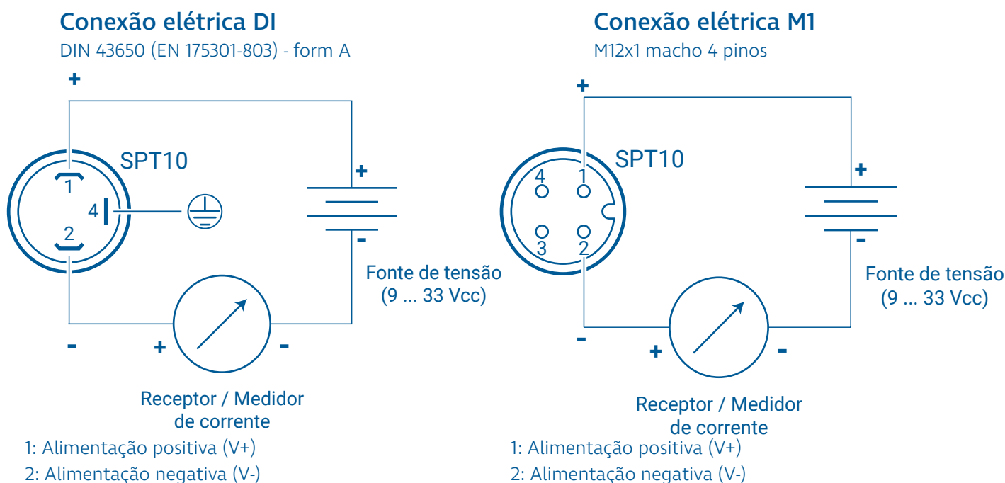
Figura 4 - Esquema de ligação 4...20 mA do transmissor SPT10
