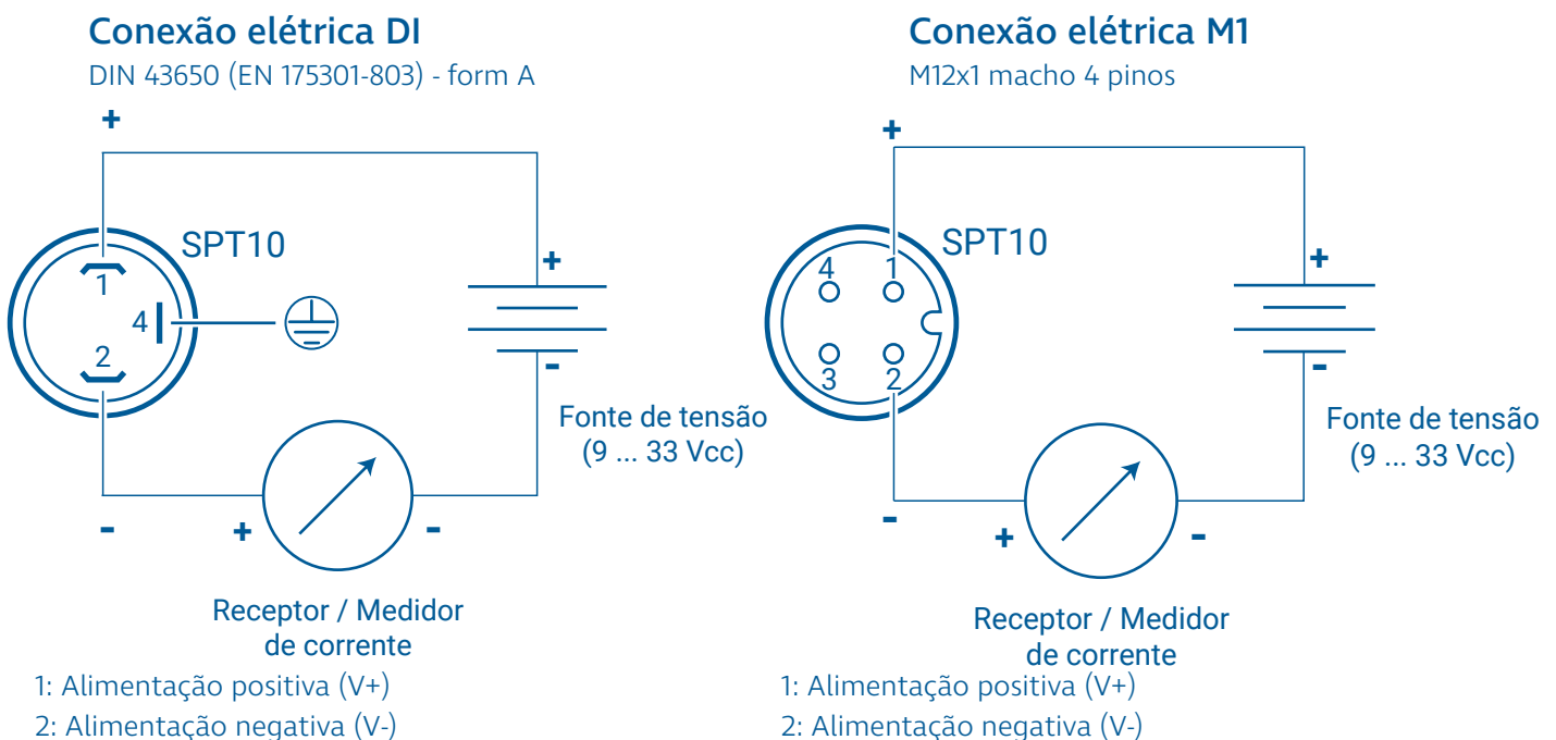
Figura 4 - Esquema de ligação 4...20 mA do transmissor SPT10
